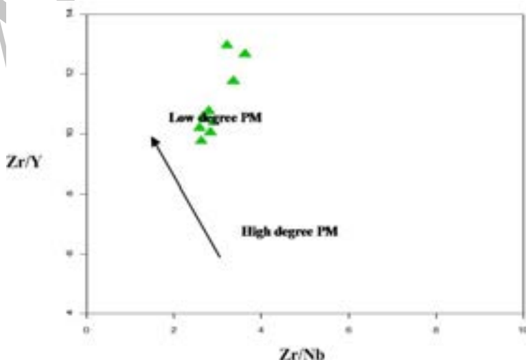
شکل ۱۳- نمودار Zr/Nb در برابر Zr/Y (Kuepouo et al. , 2006)
