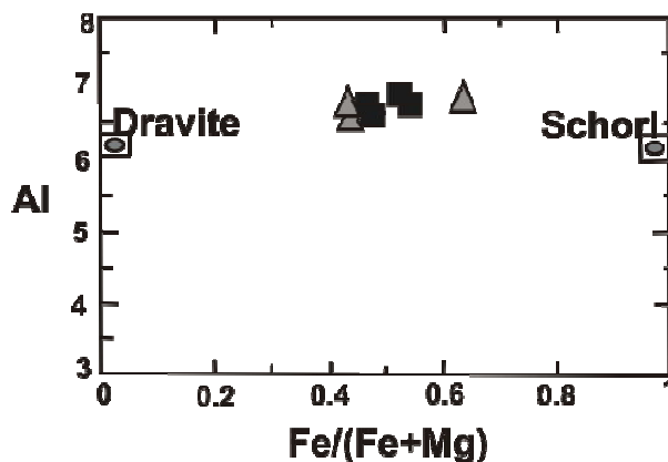
شکل ۱۰ نمودار Al نسبت به [Fe/(Fe + Mg)] و مقایسه‌ی ترکیب تورمالین های چاه رویی با ترکیب ایده آل شورل- دراویت. نمونه‌های تورمالین چاه رویی غنی از آلومینیم. نشانه‌ها مانند شکل ۸.
