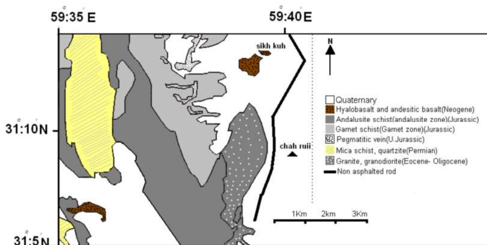
شکل ۲ نقشه‌ی زمین شناسی منطقه‌ی چاه رویی [۱].
