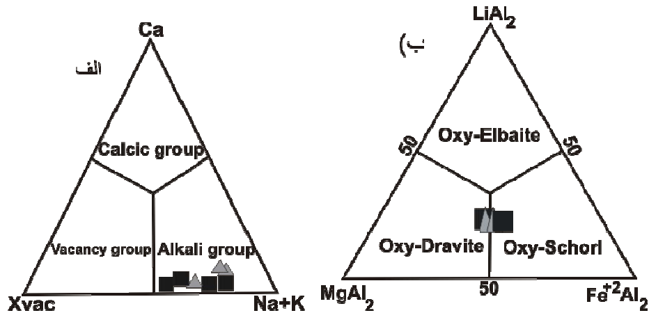
شکل ۷ الف) نمودار سه تایی [X] Xvac - Ca - Na + K زیرگروه تورمالین‌ها بر اساس قرارگیری در جایگاه X (ب) نمودار سه تایی [X] MgAl_2 - LiAl_2 - FeAl_2 زیرگروه قلیایی تورمالین‌ها بر اساس قرارگیری در جایگاه X و Y. نشانه‌ها مانند شکل ۸ ب.
