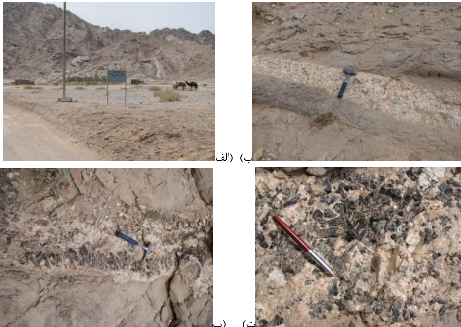
شکل ۴ عکس‌هایی از منطقه‌ی مورد بررسی. الف) نمایی از گرانیتوئید چاه روی (ب) نمایی از پگماتیت‌هایی که در درون توده‌ی گرانیتوئیدی چاه روی‌اند و دارای بیوتیت‌اند و از فراوانی کم تورمالین برخوردارند (پ) نمایی از پگماتیت‌های نوع CH که حاوی تورمالین و فاقد بیوتیت (ت) نمایی نزدیک از تورمالین در صحرا که فاقد بیوتیت است.
