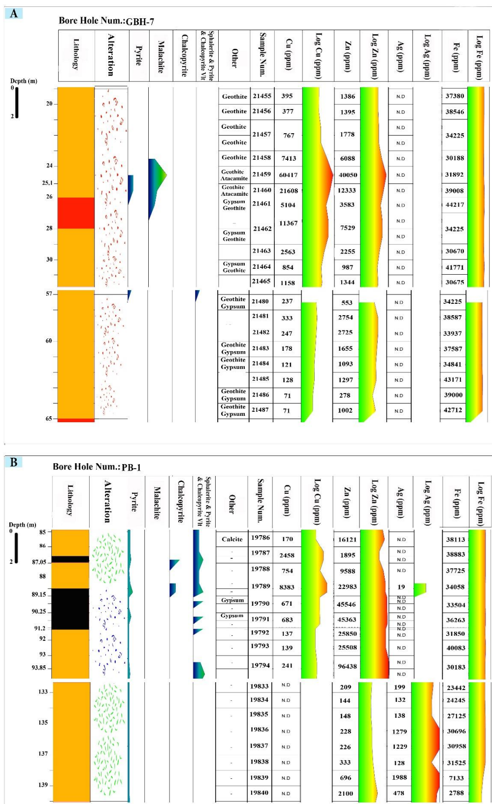
شکل 13. A: نمودار چاه‌نگاری گمانه GBH-7 (کانسار ماهور)، B: نمودار چاه‌نگاری گمانه PB-1 (کانسار ماهور) (علایم همانند شکل 12)
