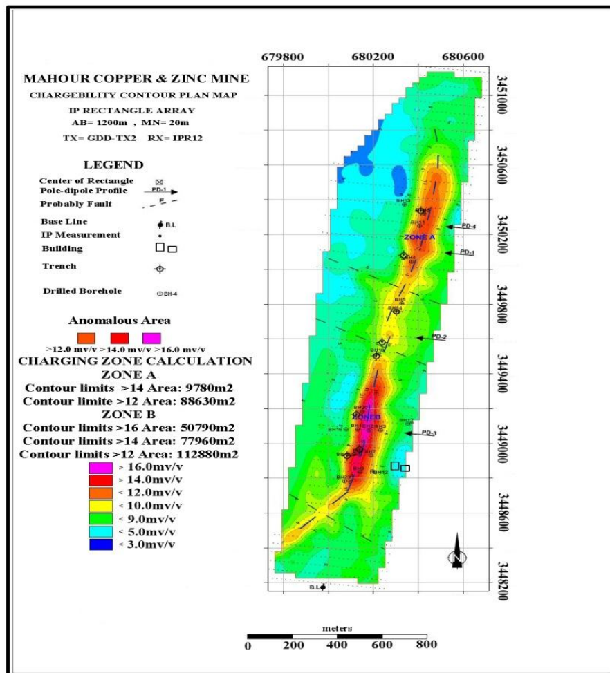
شکل 6. نقشه بارپذیری کانسار ماهور
