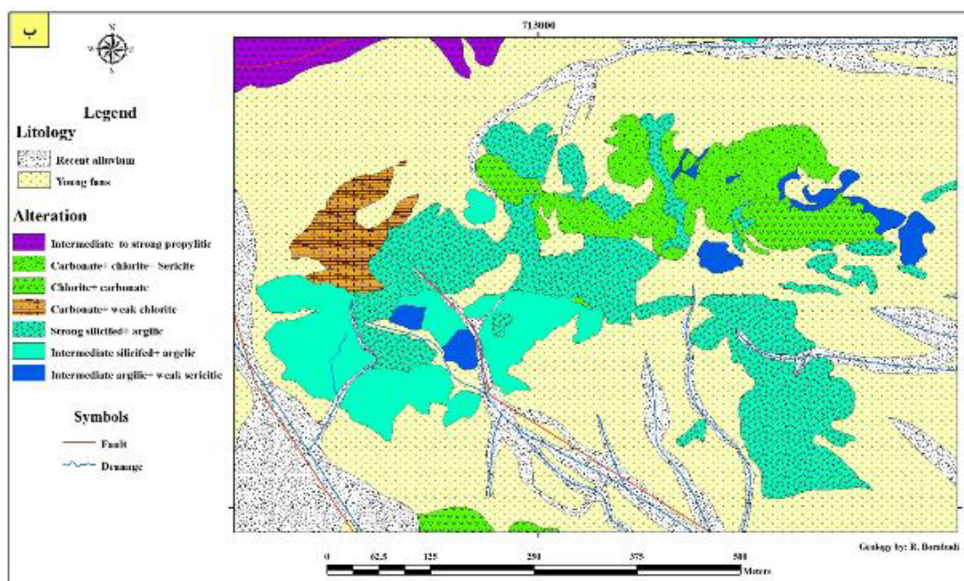
شکل ۷ نقشه‌ی دگرسانی گسترده‌ی پی‌جویی سیمرغ (الف) با مقیاس ۱:۱۰۰۰۰ (ب) با مقیاس ۱:۱۰۰۰.
