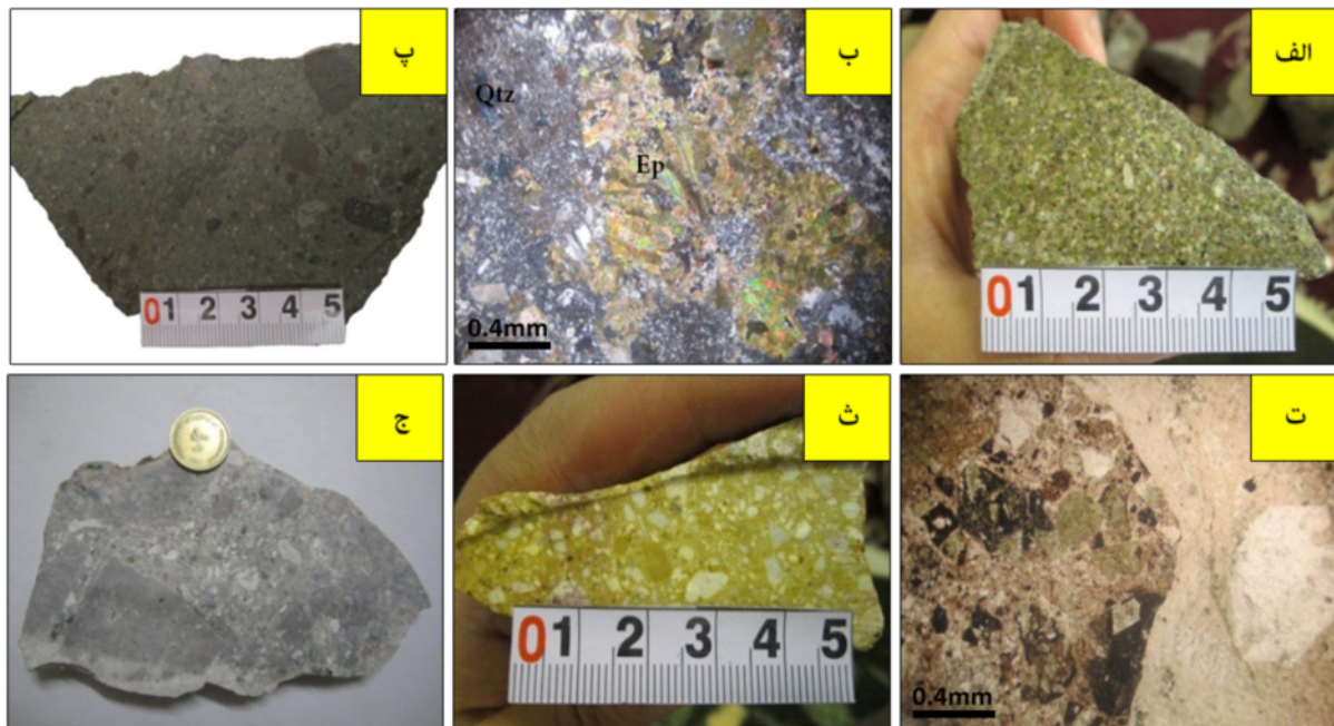
شکل ۶ الف. نمونه‌ی دستی توف برشی ب. مقطع میکروسکوپی توف برشی، نور PPL پ. نمونه‌ی دستی برش آتشفشانی ت. قطعه برشی درون آن، نور PPL. ث. نمونه دستی برش گرمایی منو مکتیک با سیمان سیلیسی و ژاروسیت ج. نمونه دستی برش گرمایی پلی مکتیک با سیمان سیلیسی. Ep: اپیدوت، Qtz: کوارتز.
