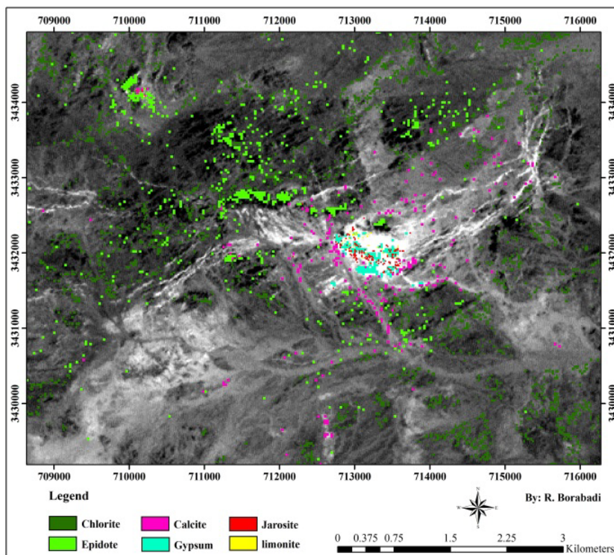
شکل ۲ پردازش تصاویر سنجنده آستر برای کانی‌های کلریت، اپیدوت، کلسیت، ژپس، زاروسیت و لیمونیت.
