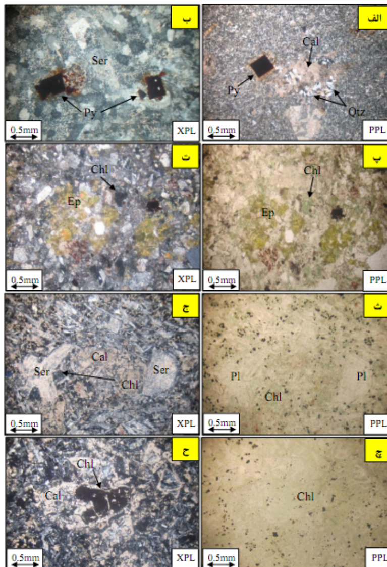
شکل ۸ الف. دگرسانی کوارتز + سرسیت + پیریت + کربنات در دایک هورنبلند گرانودیوریت پورفیری، ب. دگرسانی کوارتز + سرسیت + پیریت در دایک سینیت پورفیری، پ و ت. دگرسانی پروپلیتیک شدید در واحد توف برشی، ث. دگرسانی کربنات + کلریت + سرسیت در توده دیوریت پورفیری و ج. دگرسانی کربنات + کلریت در توده دیوریت پورفیری. Cal: کلسیت، Ep: اپیدوت، Qtz: کوارتز، Chl: کلریت، Ser: سرسیت.
