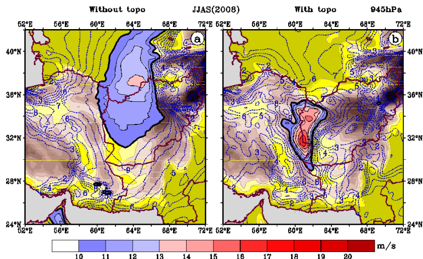
شکل (۱۲). شدت باد در شرایط با توپوگرافی (سمت راست) و بدون توپوگرافی (سمت چپ) شرق فلات ایران در تراز بیشینه سرعت باد (۹۴۵ ه.پ.). پربند سیاه پرنگ نشان دهنده سرعت باد ۱۰ متر بر ثانیه است.
