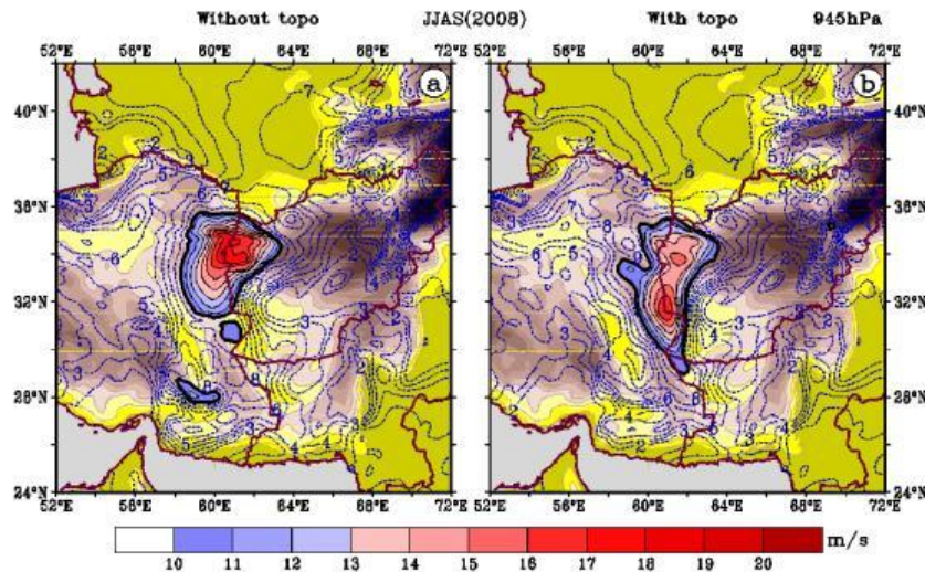
شکل (۵). شدت باد در شرایط با توپوگرافی (سمت راست) و بدون توپوگرافی خراسان جنوبی (سمت چپ) در تراز بیشینه سرعت باد (۹۴۵ ه.پ.). پرنده سیاه پرنده نشان دهنده سرعت باد ۱۰ متر بر ثانیه است.
